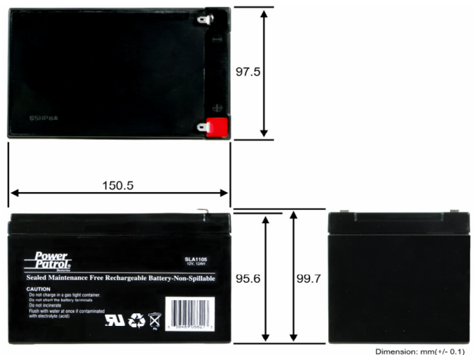
Dimension: mm(+/- 0.1)
